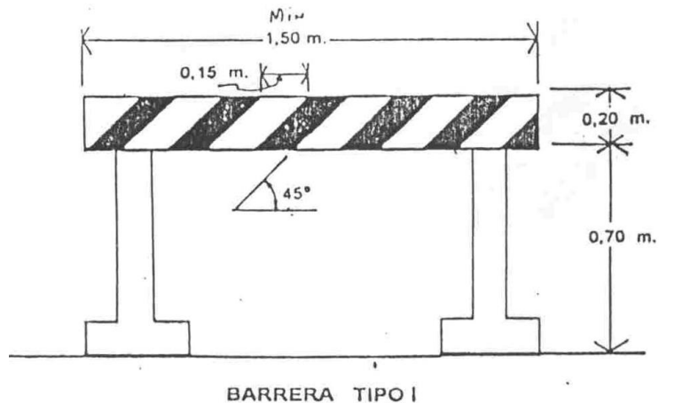
BARRERA TIPO I
