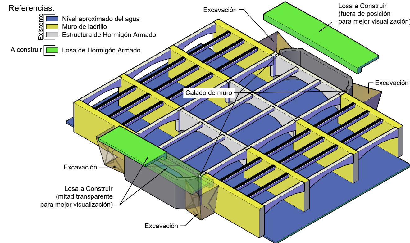
Axonometria esquemática de subestructura esc:S/E
