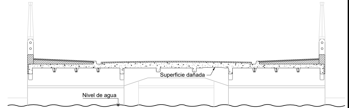
Sección A-A' esc:1/100 (Niveles aproximados)
