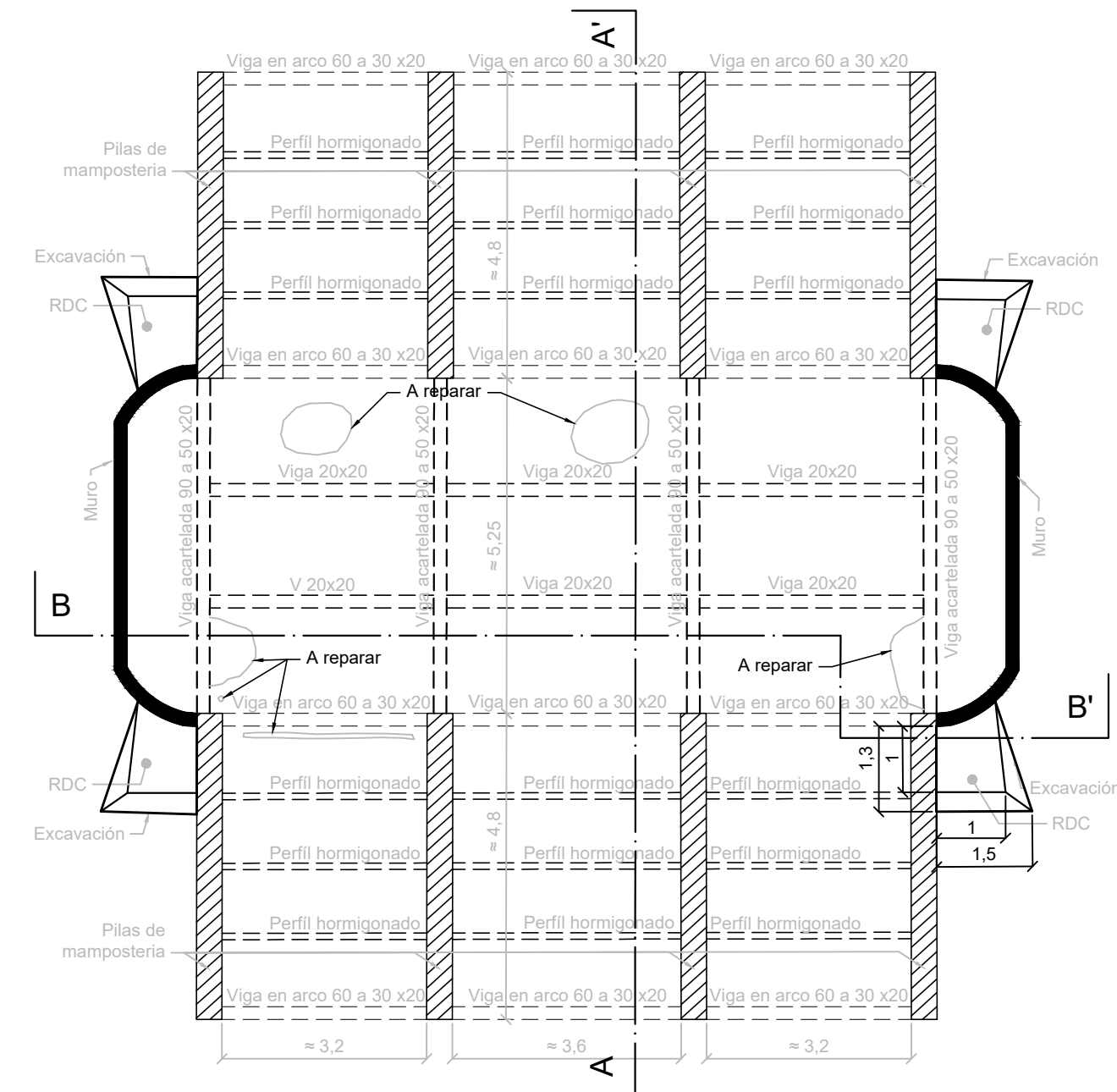
Subestructura esquemática esc:1/100 (Medidas aproximadas)
