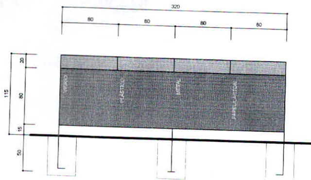
VISTA POSTERIOR
