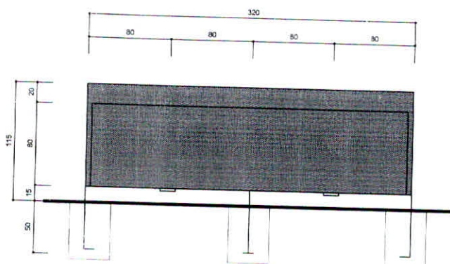
VISTA POSTERIOR
