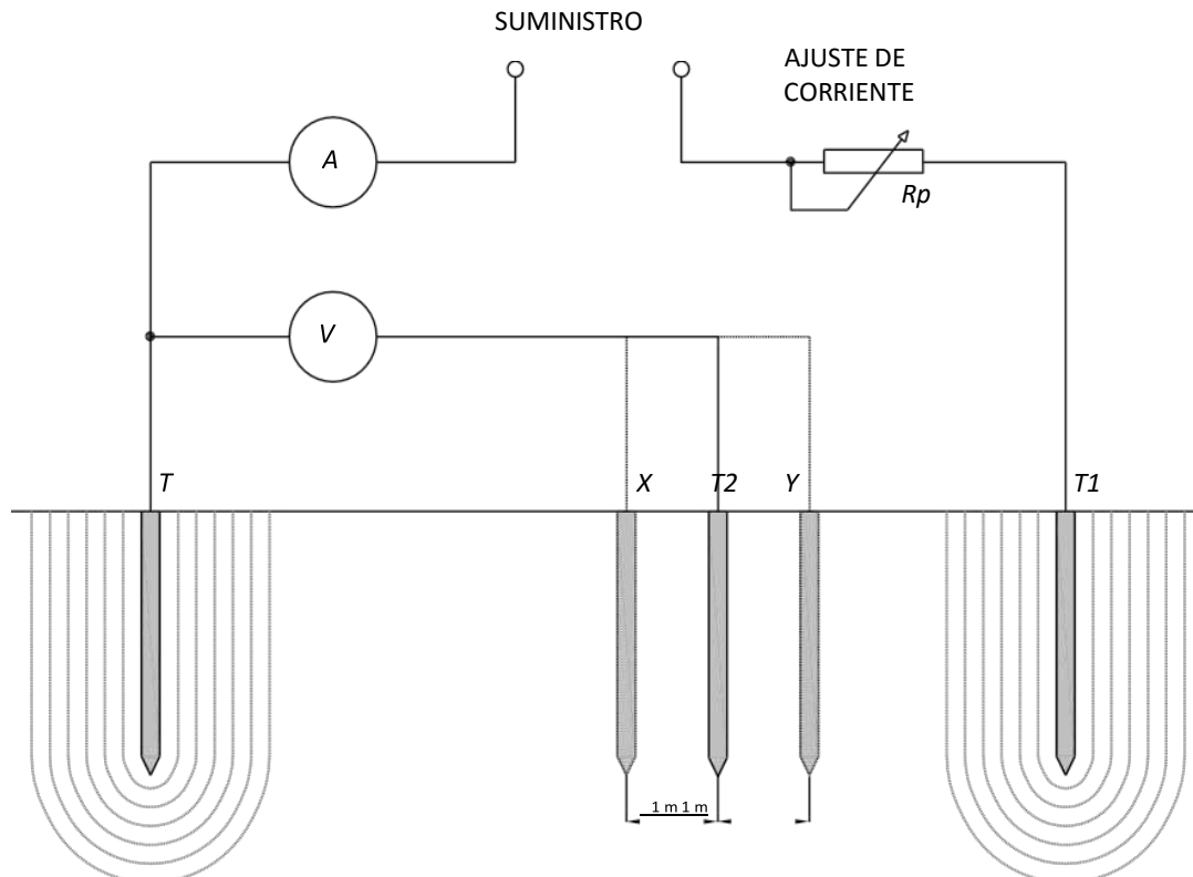
Figura 770.19.A – Método para la medición de resistencia de puesta a tierra
