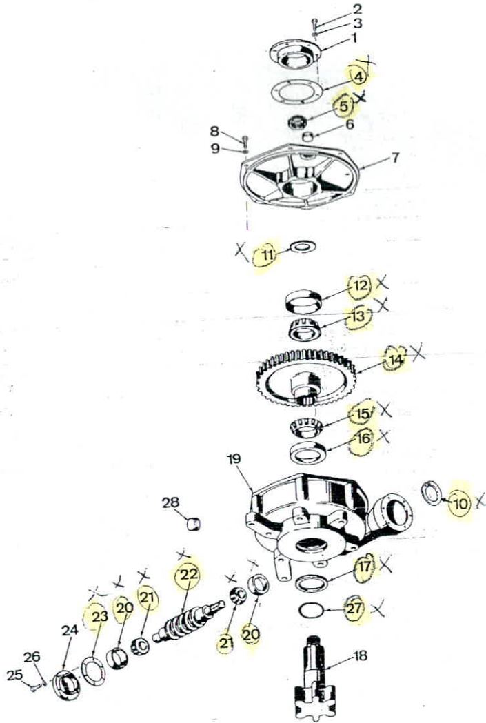
FIG. 17100 REDUTOR DO CÍRCULO 1 Circle Reserve, Gear case Reductor del Círculo
