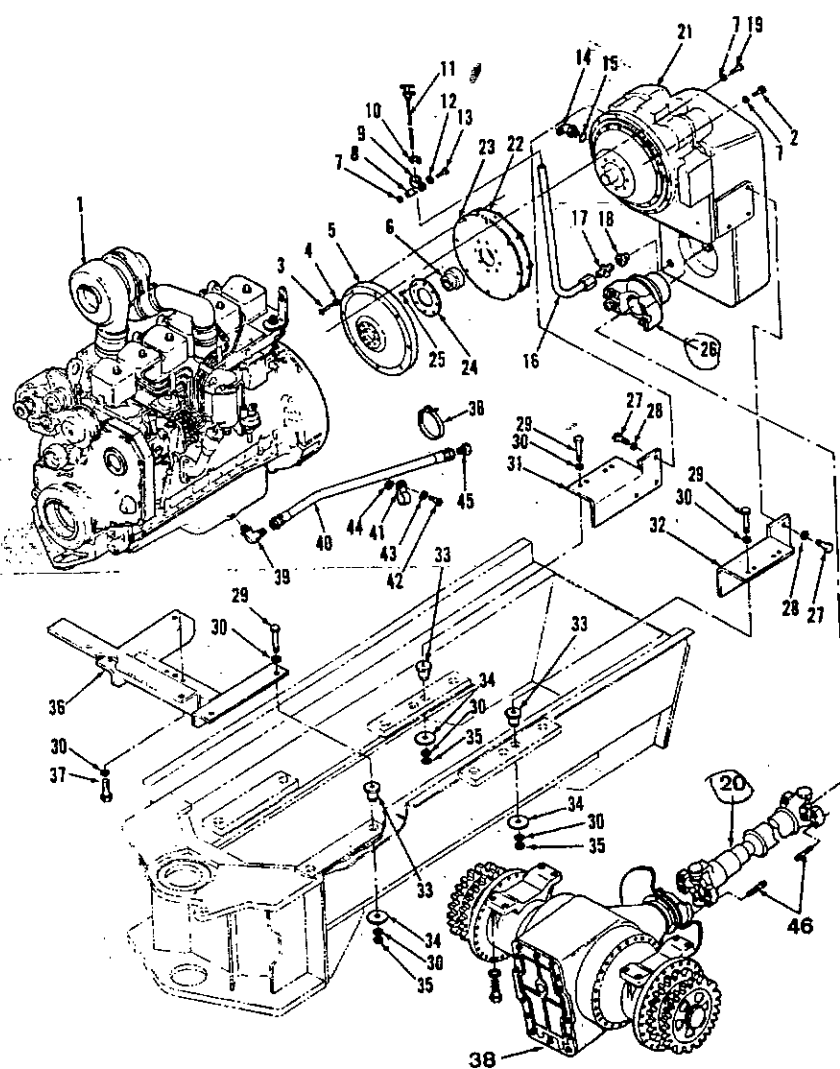
FIG. 7020 SISTEMA MOTRIZ Drive Line Línea Motriz
