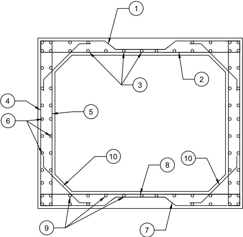
DISTRIBUCION DE ARMADURAS
