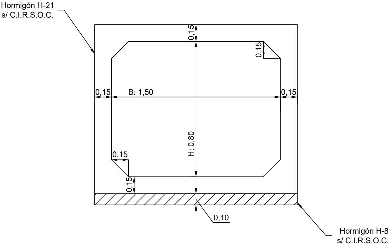
SEMI-SECCIÓN TRANSVERSAL
