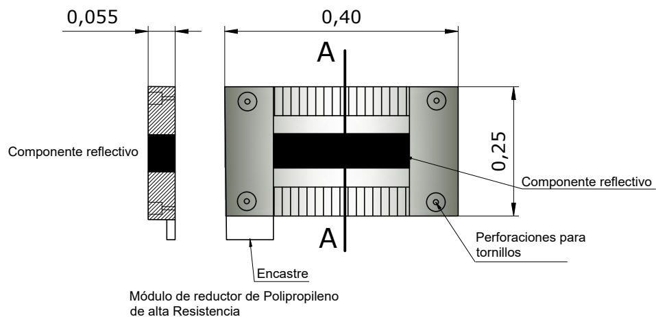
Corte AA
