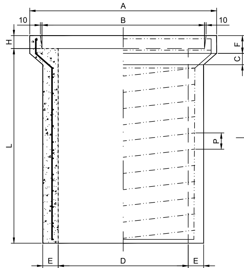
SEMI-CORTE LONGITUDINAL
