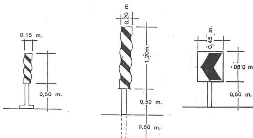
DELINEADORES
