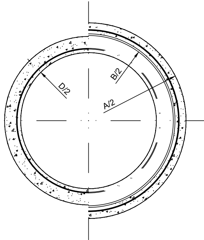
SEMI-CORTE TRANSVERSAL
