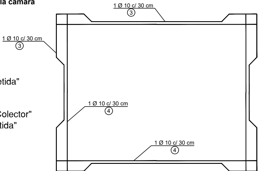
Detalle Caño
