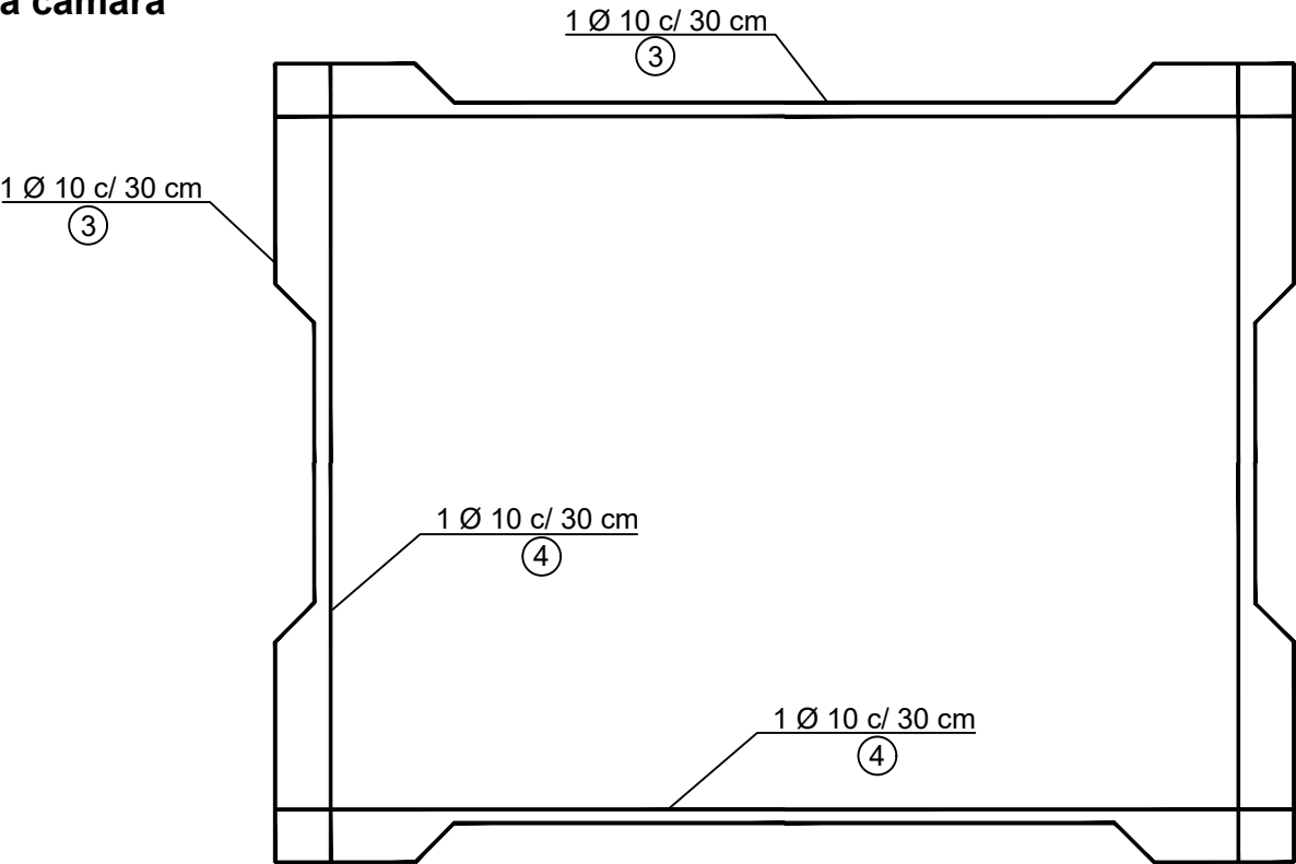
Detalle hierros horizontales de la cámara
